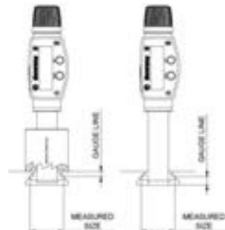
Autres mesures de fentes en queue d'aronde et conique
